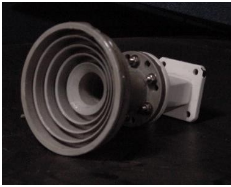
Antena de bocina coarrugada
