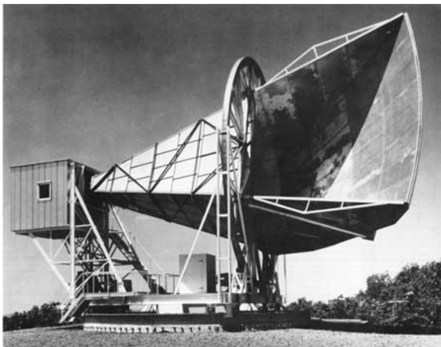
Antena de bocina (año 1960)
