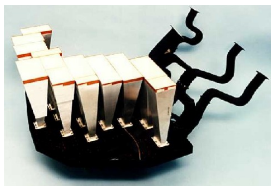
Agrupaciones de antenas ranuradas y de antenas de bocina
